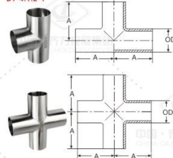
中卡式等径短三通 Weld/Clamp Tee
