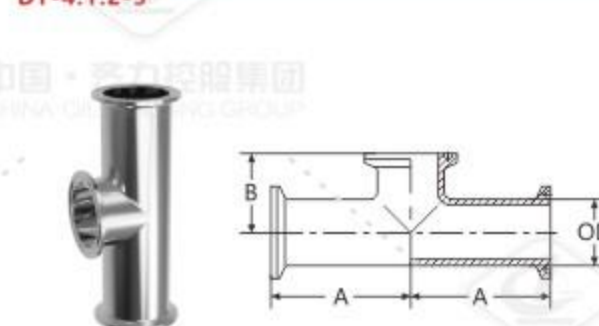
卡式等径短三通 Clamp Tee
