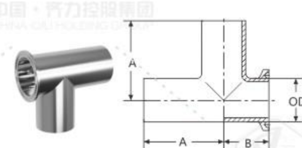
一端卡式等径短三通 Weld/Clamp Tee
