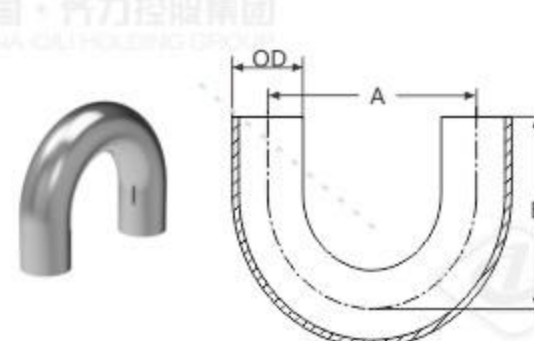
180°长弯头 Weld 180° Long Bend
